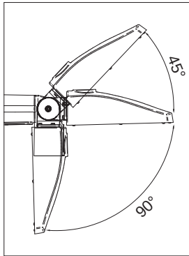
Oszlopfejre vagy oszlopkarra (állítható nyaköntvénnnyel)
