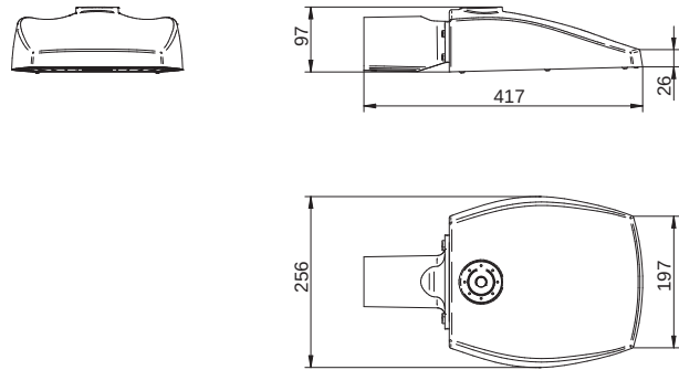
TWINI FIX NYAKÖNTVÉNNYEL
