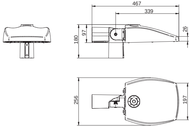
TWINI ÁLLÍTHATÓ NYAKÖNTVÉNNYEL
