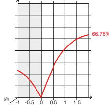
Lámpatest dőlésszög 0°
